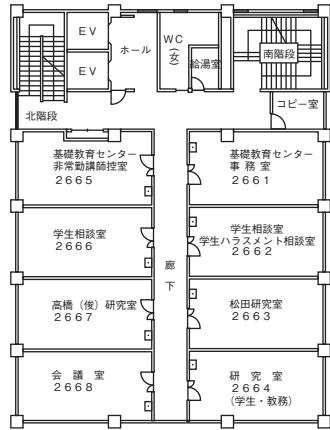
6階 平面図
